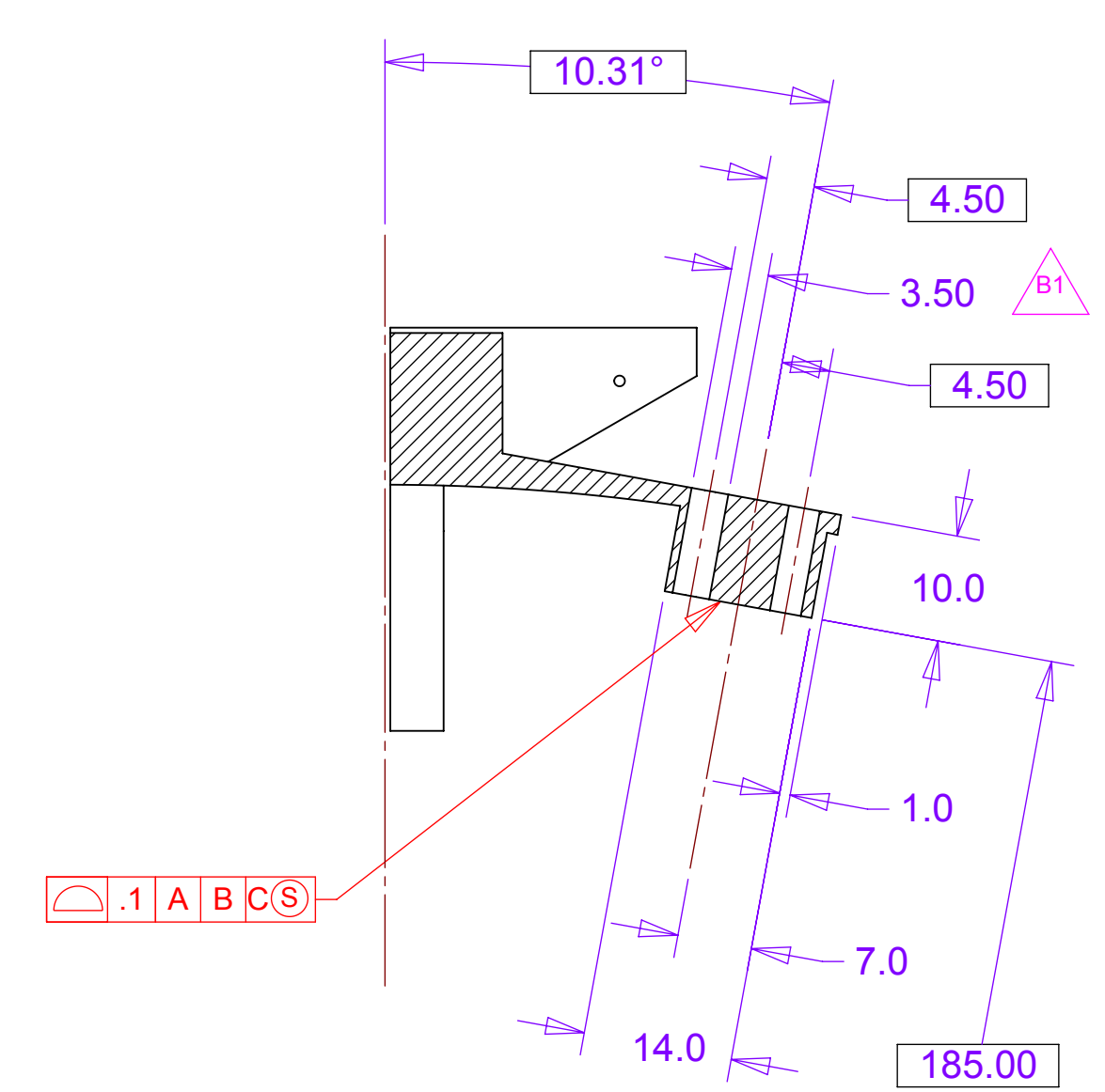
SECTION D-D
