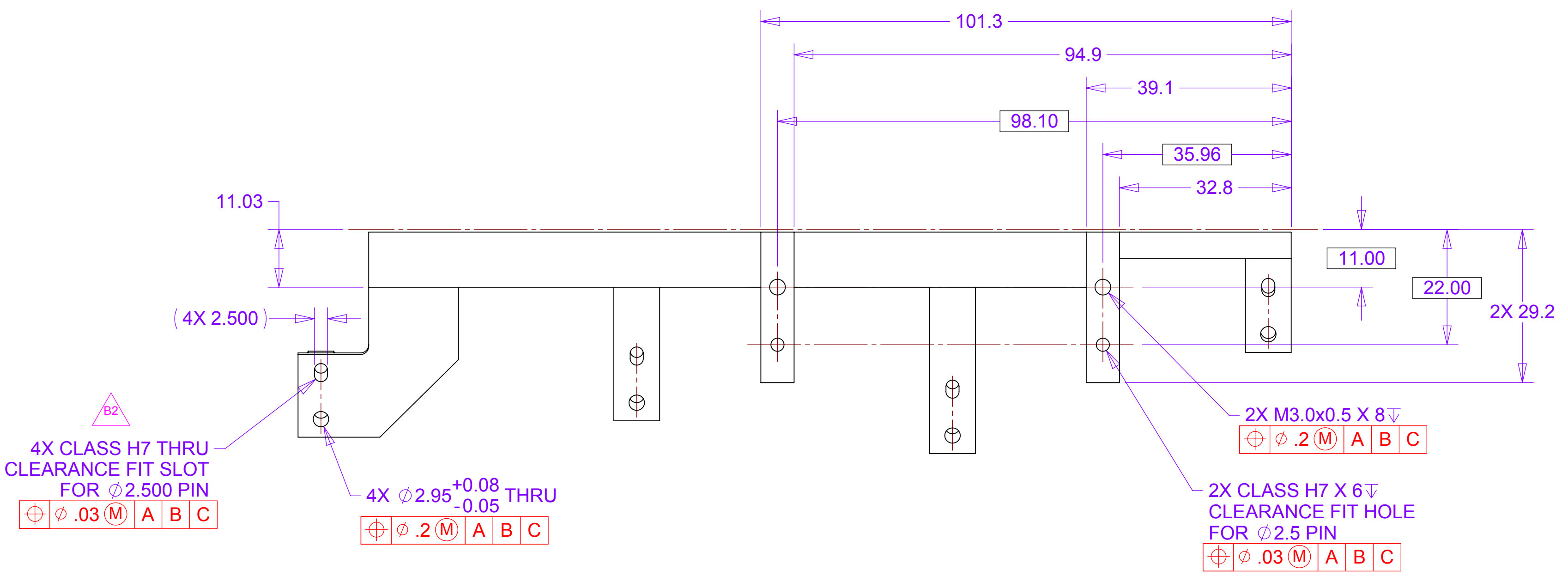
SECTION A-A
